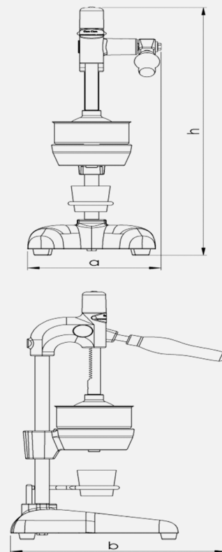
Чертеж 1
